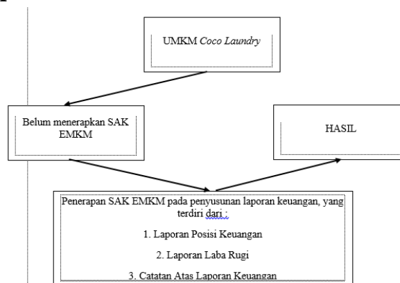
Gambar.1 Kerangka Berpikir
